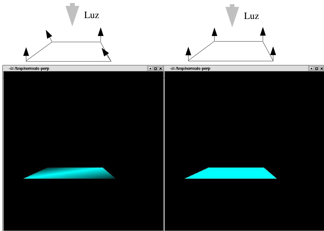
Figura 5.1. Efecto de las normales en la iluminación
