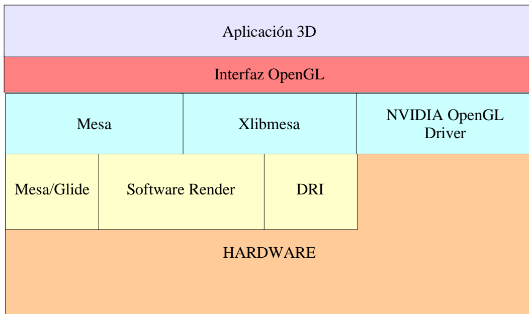
Figura 2.1. Acceso al hardware a través de OpenGL (Linux)
